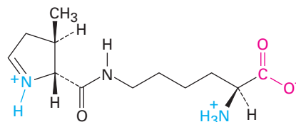
Pyrrolysine
