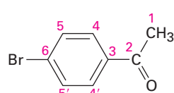
para -Bromoacetophenone
