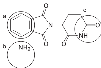
Pomalidomide
