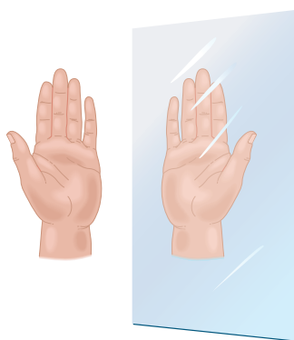
Left hand
