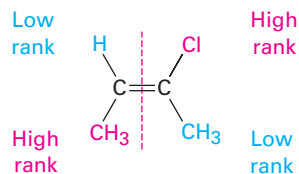
(a) ( E )-2-Chloro-2-butene
