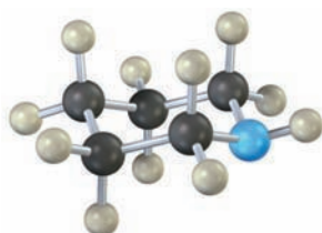
Piperidine
