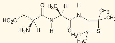
Alitame
