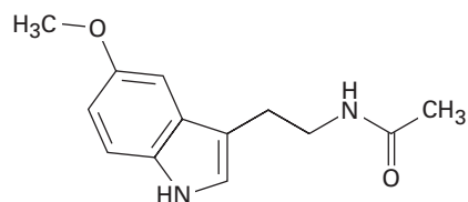
Melatonin
