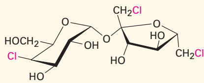
Sucralose
