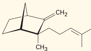
\beta -Santalene (sandalwood oil)
