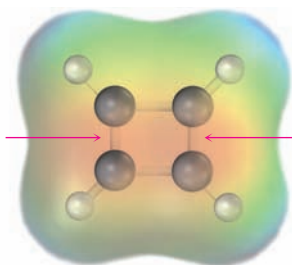
Cyclobutadiene
