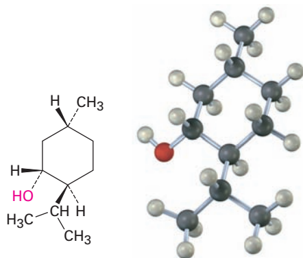
Menthol
