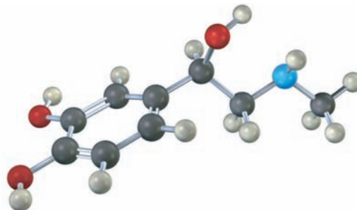
Adrenaline
