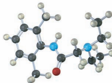
Lidocaine
