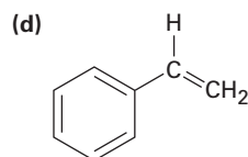
Styrene
