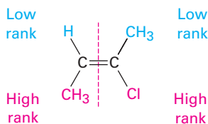
(b) ( Z )-2-Chloro-2-butene
