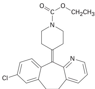
Loratadine
